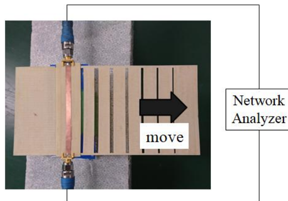
図 6: 試作品と実験環境
