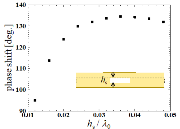
図2：スリット厚 h_s と位相変化量の関係
