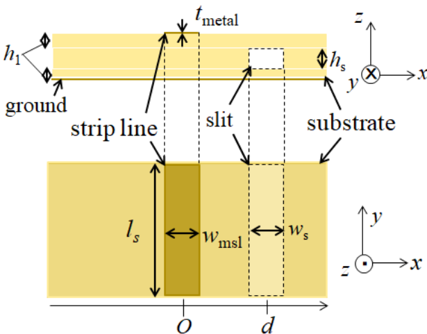
図1：提案移相器の構造 ( w_{msl} = 0.16\lambda_0 , l_s = 2\lambda_0 , h_1 = 0.012\lambda_0 )
