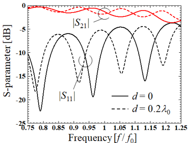
図 4: 提案移相器の S パラメータ
