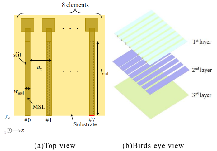
図 8: 提案移相器を有するアンテナアレー
